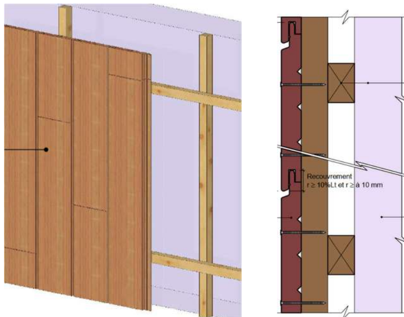
Figure 4 : Lames à emboîtement – pose verticale (illustration 3D et coupe horizontale)
